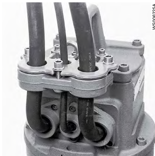
Рис. 15: Держатель кабеля. В насосах с MAS 801 нет вспомогательного кабеля.
