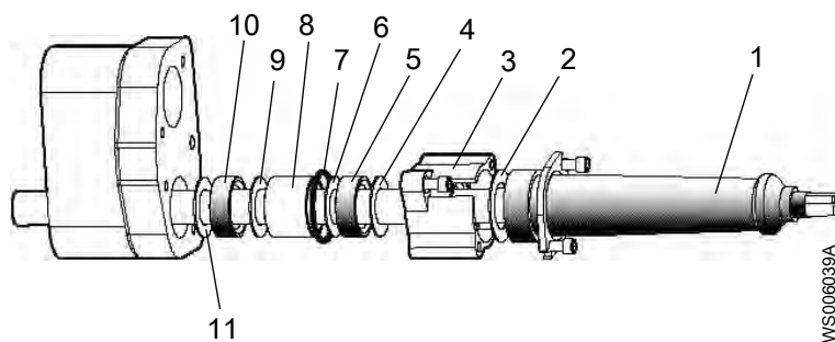
Рис. 10: Блоки привода 605–675
