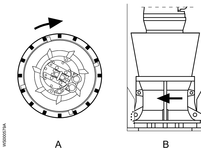
Рис. 28: Вид сверху (А) и вид сбоку (В)
