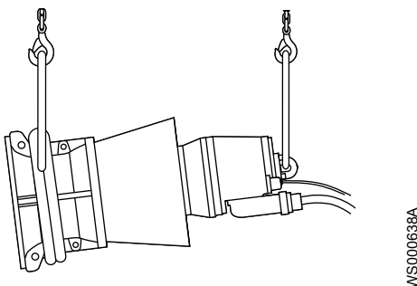
Рис. 30: Поднимите агрегат для ремонта. Показан типовой агрегат.
