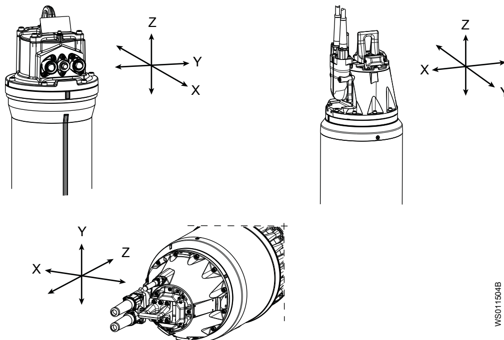
Рис. 4: Направление вибрации по отношению к насосу
